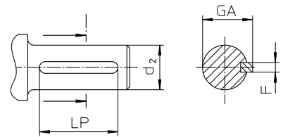
Einzelheit X / Detail X / Détail X M 1:5
